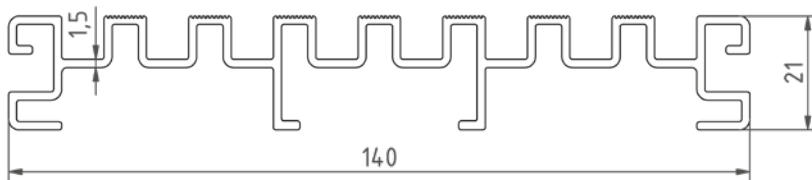
Seitenansicht
